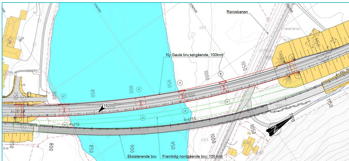
Figur 6: Ny Gaula bru på vestsiden av eksisterende bru – utsnitt fra teknisk plan. Kilde: Norconsult.
